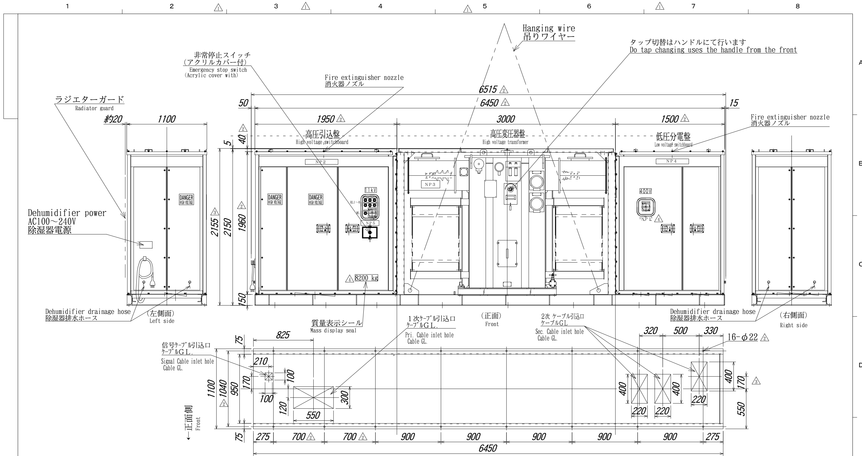
(ケース上面から見たベース詳細図) Base detail drawing from the case upper side
