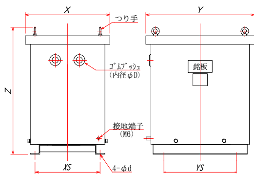
◎ 屋内防滴ケース入
