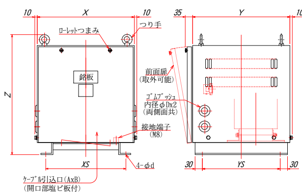
◎ 屋内通気ケース入
