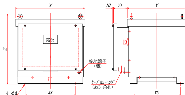
◎ 屋外防雨ケース入
